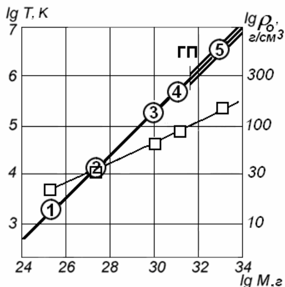
Рис. 8-5. Температура T образования звезд (Солнце - 5), Коричневого Карлика (4), Юпитера (3), Земли (2) и Луны (1) как функция их массы M . Плотность центральной части тел (квадраты) в момент их образования.
