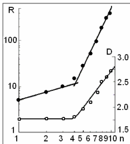
Рис. 8-2. Зависимость расстояния планеты от Солнца R (а.е.) величины фрактальной размерности D от порядкового номера планеты n ( \lg-\lg ). 1- Меркурий, 2- Венера, 3 – Земля, 4 – Марс, 5 – пояс астероидов, 6 – Юпитер и т.д.
