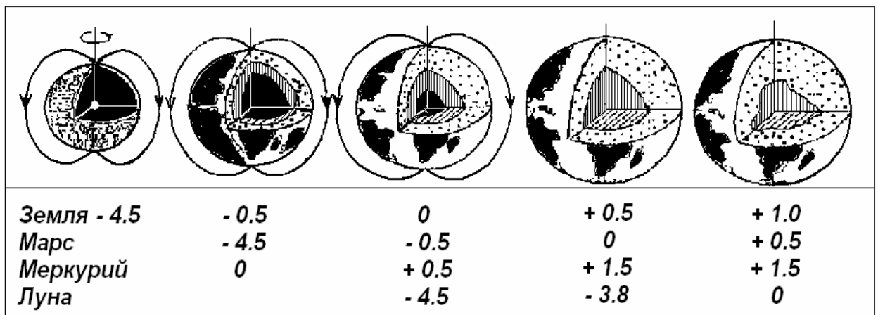
Рис. 8-6. Внутреннее строение Земли, Марса, Меркурия и Луны на различных этапах эволюции.
