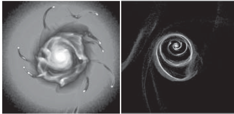
Рис. 8-1. Расчеты на суперкомпьютере (Снытников и др., 2002). Слева: сгустки вещества при развитии гравитационной неустойчивости. Справа: кольцеобразные структуры из частиц твердой фазы. Количество частиц в расчетах - 300 000.
