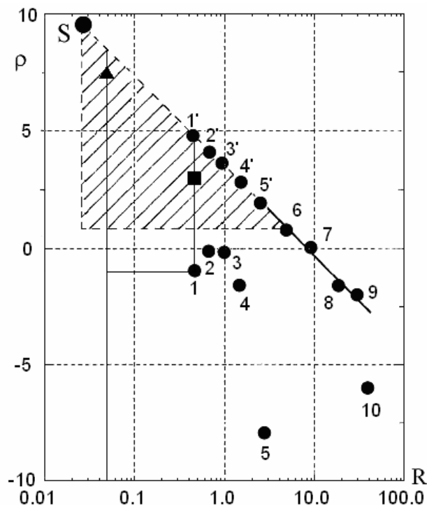
Рис. 8-3. Величина поверхностной плотности для планет Солнечной системы (lg-lg). Масса заштрихованного треугольника равна массе Солнца. Объяснения – в тексте.
