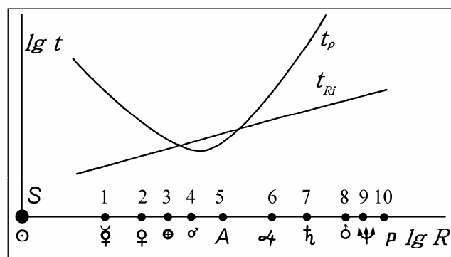
Рис. 8-4. Соотношение ( \lg - \lg ) времён образования планеты t_p и стягивания вещества кольца t_R в зависимости от расстояния планеты R до Солнца (S). 1 – Меркурий, 2 – Венера, и т.д.
